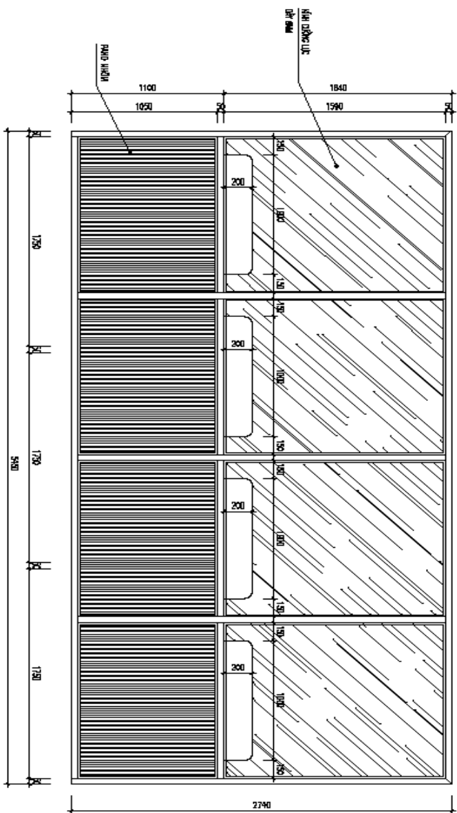
MẶT BẰNG VÁCH QUẦY ĐÓN TIẾP - SÀN CHÍNH
