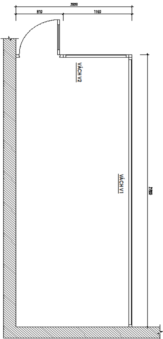
MẶT BẰNG VÁCH QUẦY ĐÓN TIẾP - SÀN CHÍNH
